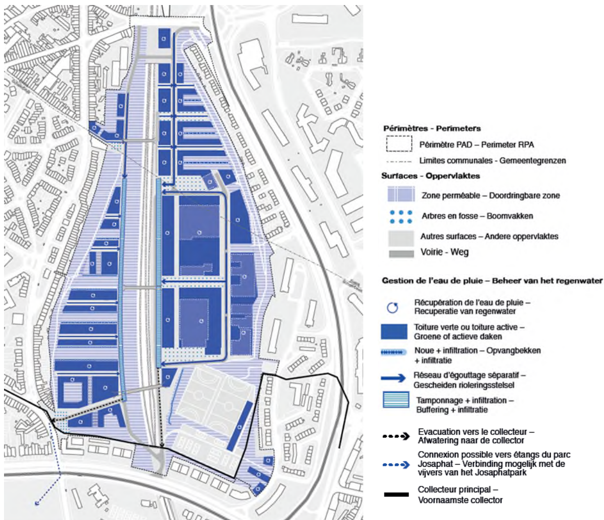
Figure 10 : Plan de gestion de l'eau du projet de PAD 2019 (MSA, 2019)
