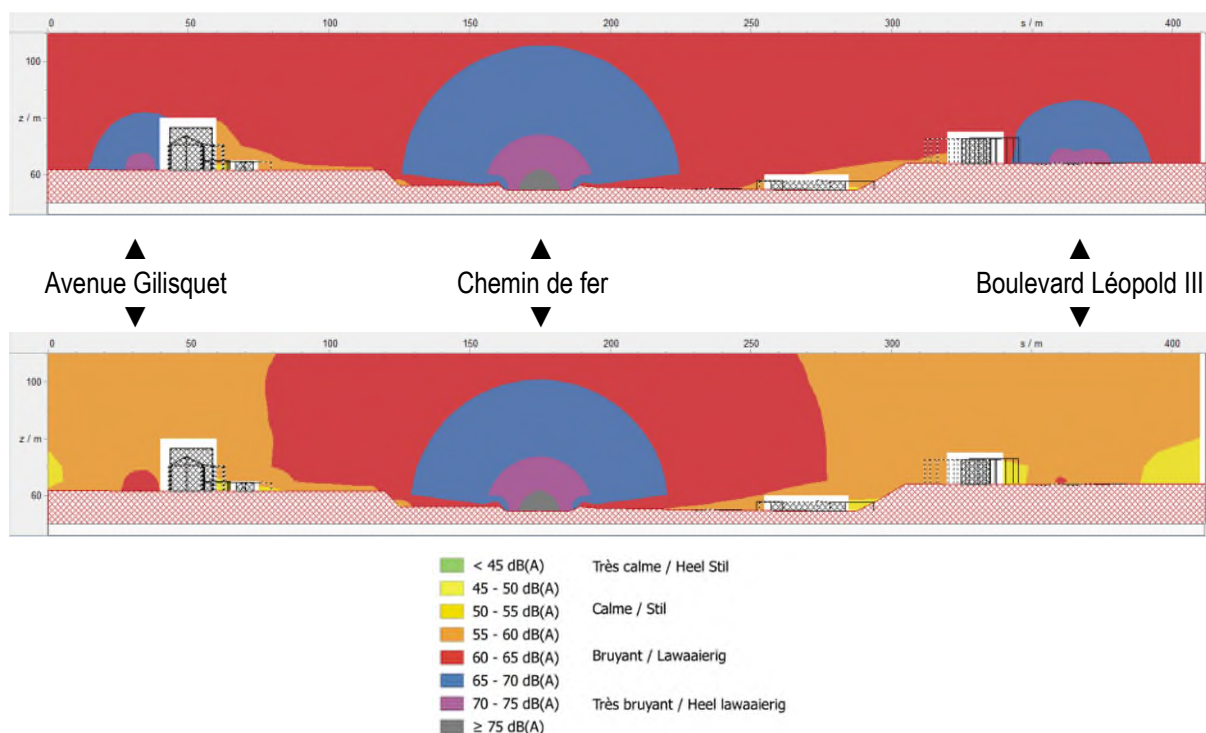
Figure 172 : Coupe de bruit A-A : passage d'un train, en période de journée (en haut) et de nuit (en bas) – Situation existante (ARIES, 2021)
