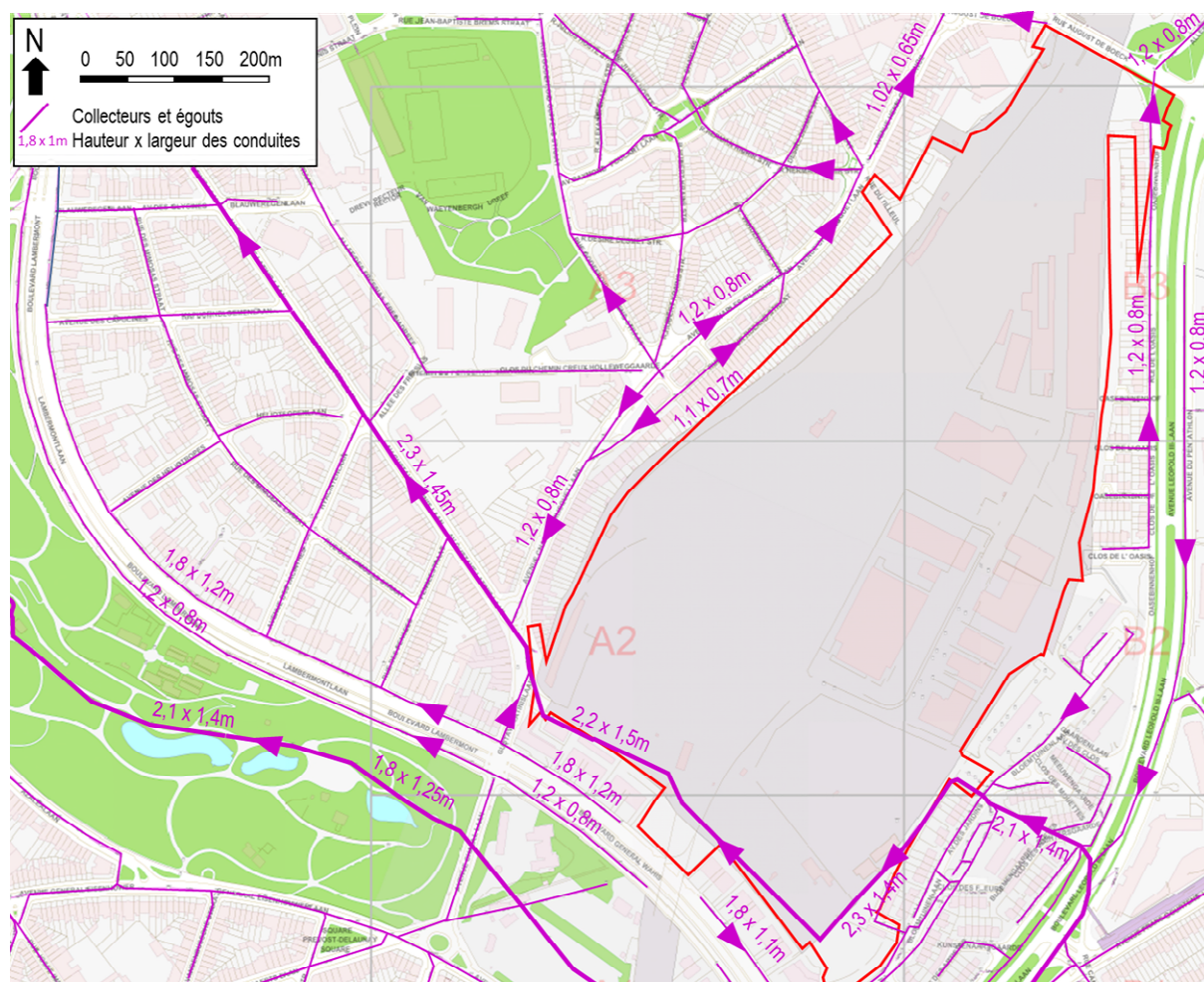
Figure 125 : Réseau d'égouttage public à proximité du périmètre du PAD (VIVAQUA, 2021)
