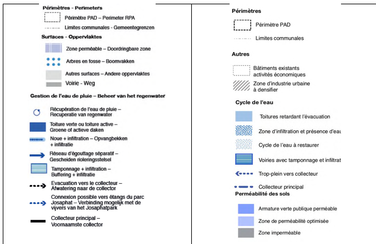
Figure 32 : Cartes de la gestion de l'eau (MSA, 2019 & 2021)
