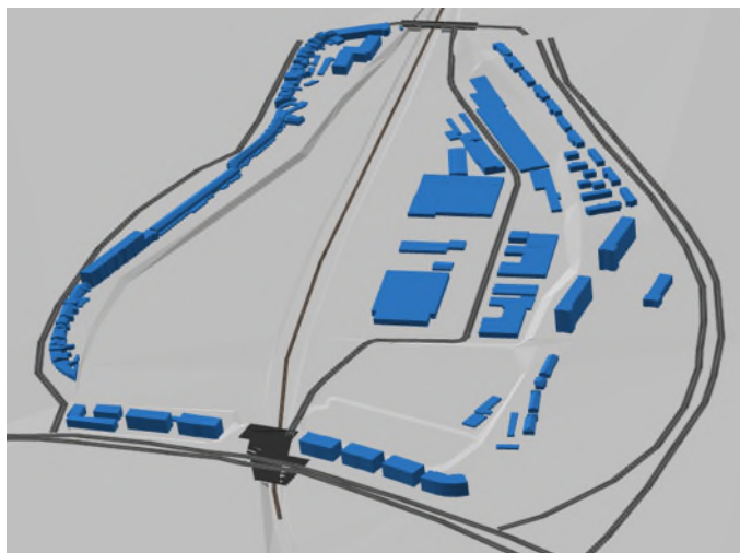
Figure 167 : Modèle 3D de la situation existante actualisée, utilisé dans la modélisation dans le logiciel IMMI (ARIES, 2021)
