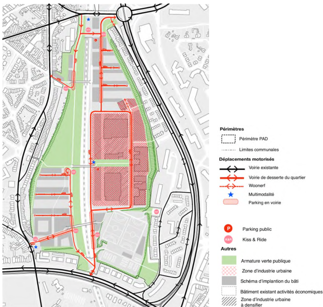
Figure 21 : Carte de la circulation automobile du projet de PAD modifié 2021 (MSA, 2021)
